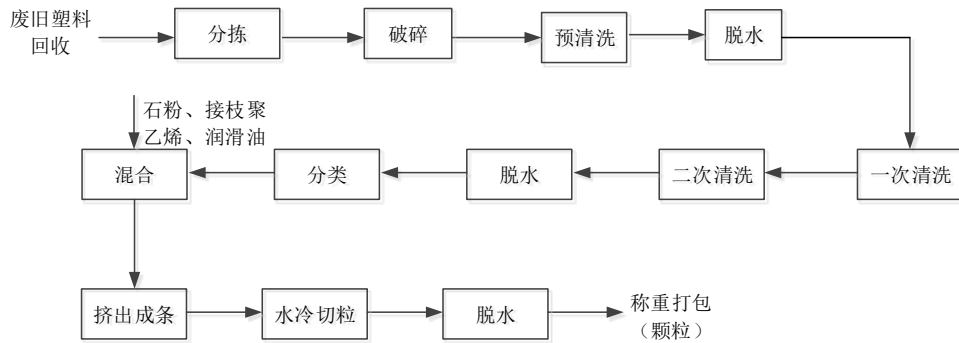
改性塑料粒子生产工艺流程图
