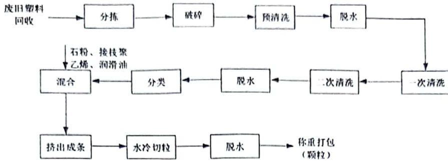
改性塑料粒子生产工艺流程图
